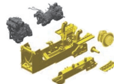
Conception modulaire de la chaîne cinématique
